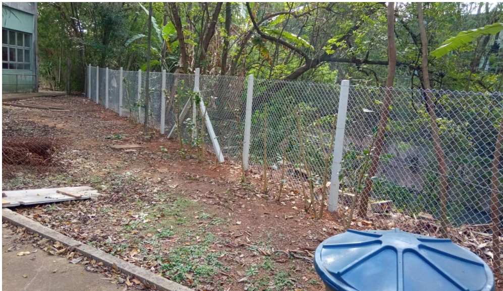
Instalação do novo alambrado na horta da Escola de Aplicação, adequação dos corrimãos e guarda-corpos das escadas e instalação de novos lavatórios
